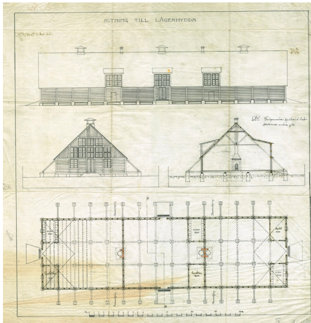
Arkitekt Erik Josephsons typritning över Lagerhydda. Fotokopia.
